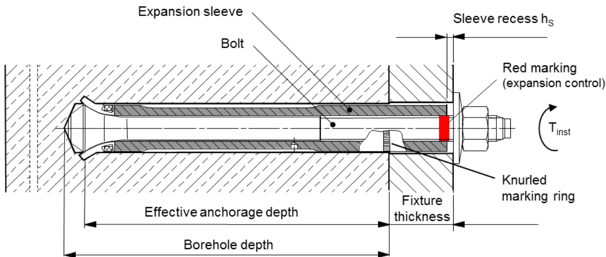
Figure A2: Version post-positionnée HDA-T et HDA-TR (Post positionnement)
