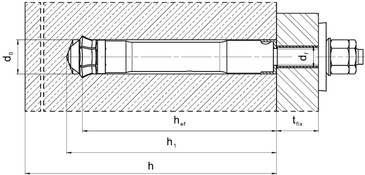
Figure A3: Version pré-positionnée HDA-P et HDA-PR (Pré-positionnement) avec kit de remplissage
