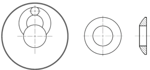
Podkładka sferyczna
