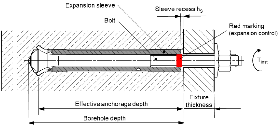
Figure A2: Version post-positionnée HDA-T et HDA-TR (Post positionnement)
